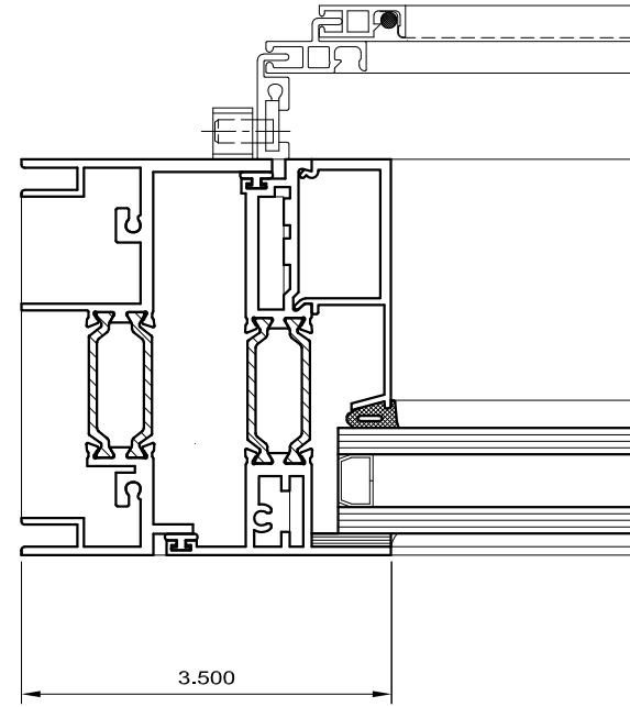
3 LEFT JAMB
