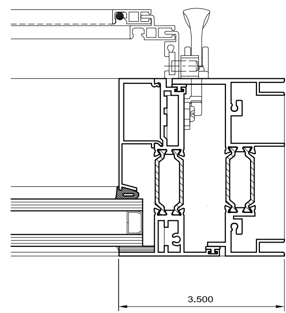
4 RIGHT JAMB
