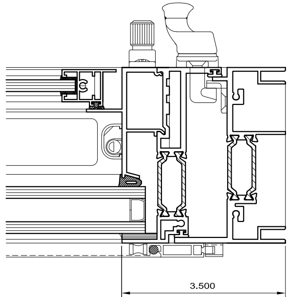
4 RIGHT JAMB
