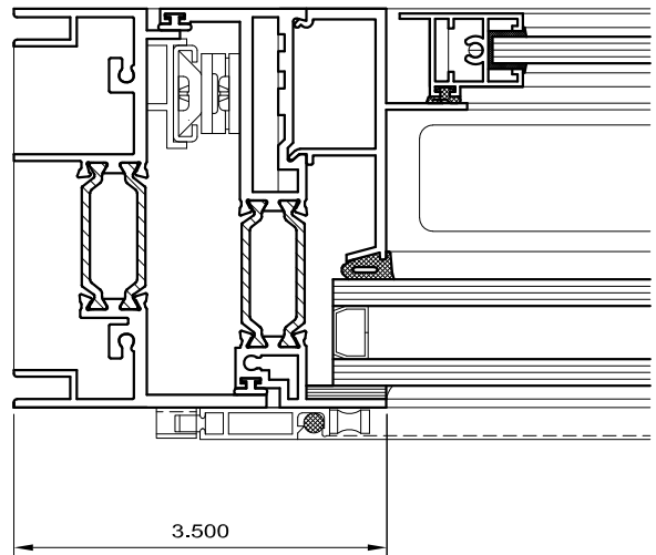
3 LEFT JAMB
