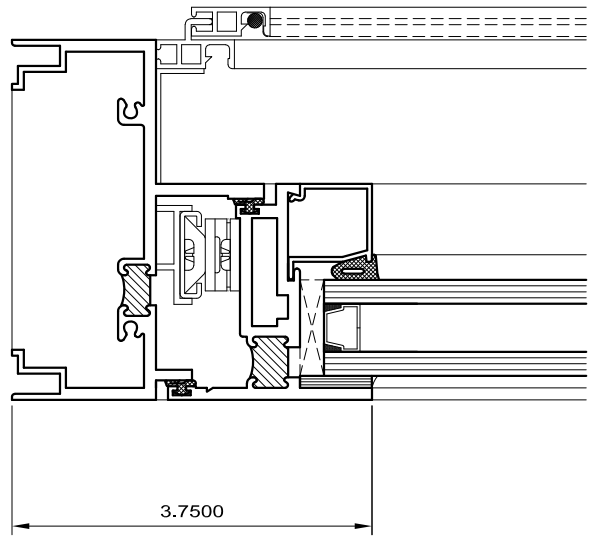
3 LEFT JAMB
