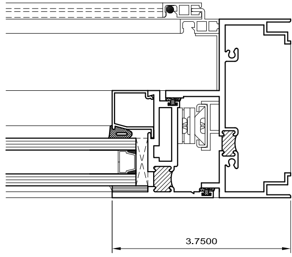
4 RIGHT JAMB
